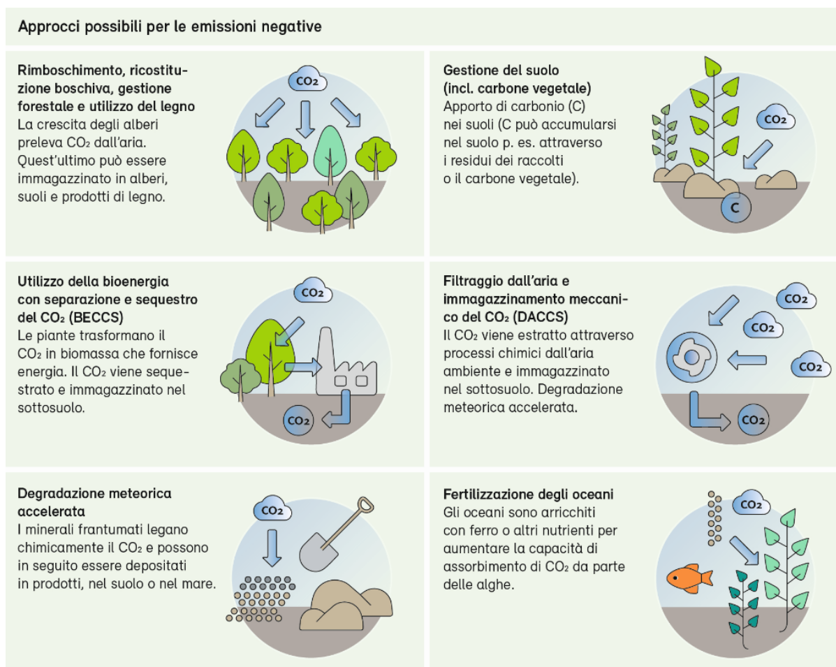
Figura 2 - Diversi approcci consentono di sottrarre CO 2 dall'atmosfera. Fonte: rappresentazione dell'UFAM basata sul Mercator Research Institute on Global Commons and Climate Change (MCC).
