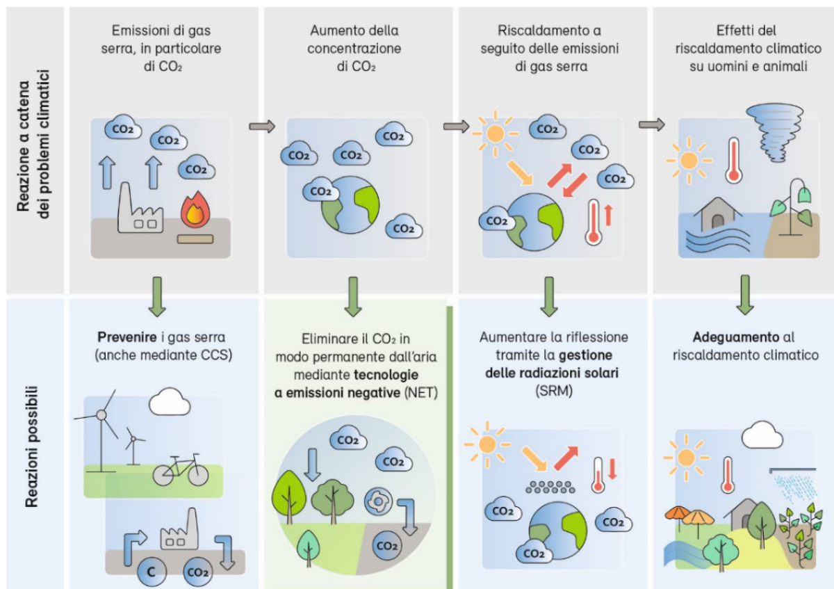
Figura 1 – Lungo la catena degli effetti del problema climatico, gli esseri umani possono reagire in modo diverso. Fonte: rappresentazione dell'UFAM basata su Jan C. Minx et. al., 2018. 2
